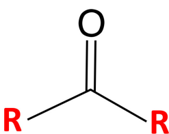
Ketone
