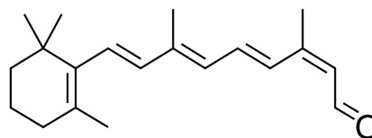
Cis-retinal
